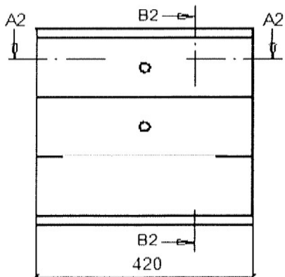
Modul SK3
