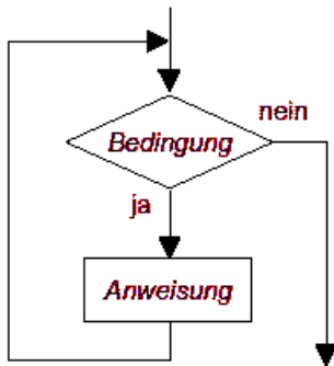
Kopfgesteuerte Schleife
