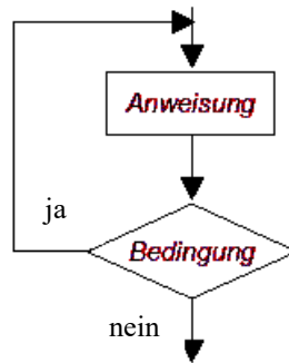
Fußgesteuerte Schleife
