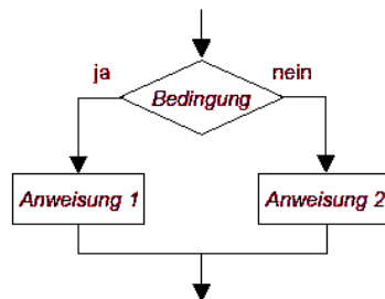
Verzweigungsanweisung
